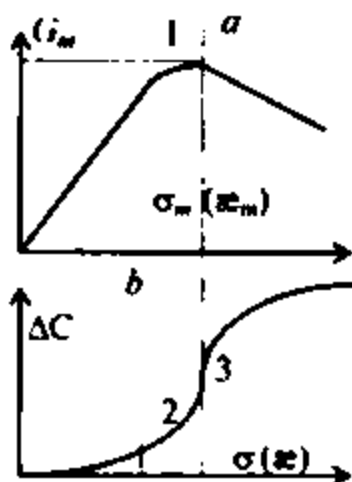
24.14-chizma. O'tkazuvchanlik aktiv qismining (a) va bo'g'in sig'iminining (b) elektr o'tkazuvchanlikka bog'liqligi. 1-past o'tkazuvchanlik sohasi; 2-sinish nuqtasi; 3-o'rta nuqta
