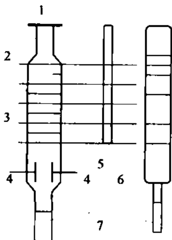
22.8-chizma. Gaz kulonometrining tuzilishi: 1-kran; 2-elektrolitik bo'g'in; 3-termostat; 5-termometr; 6-byuretka; 7-tutash shlang
