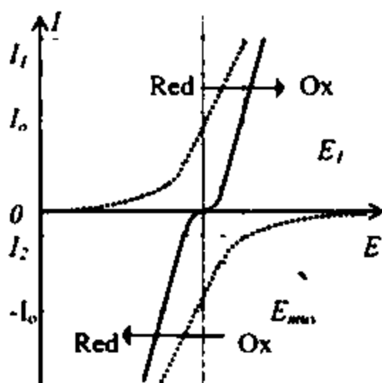
20.6-chizma. Qaytar sistemaning voltamper egri chizig'i
