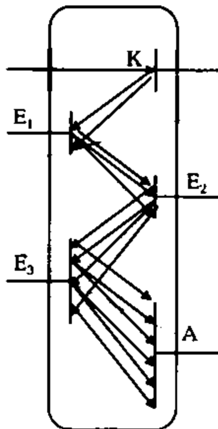
25.12-chizma. Fotoko'paytirgichning tuzilishi. K-katod; E 1 , E 2 , emitterlar. A-anod
