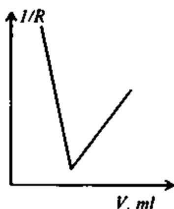
24.4-chizma. Kuchli kislotani ishqor eritmasi bilan titrlash egri chizig'i
