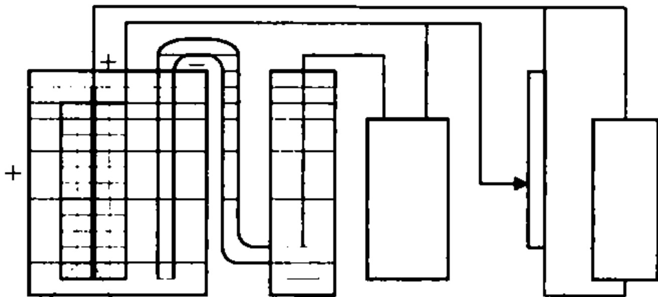
1 2 3 4 5 6 22.21-chizma. Platina elektrodida elektroliz qilish asbobining tuzilishi:
