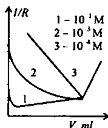
24.6-chizma. Sirka kislotaning turli xil konsentratsiyali eritmalarini titrlash
