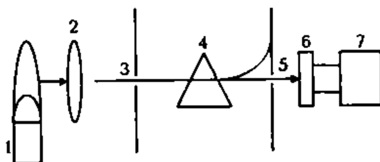
26.2-chizma. Alanga fotometrining tuzilishi: 1-gorelka (gorelkaga yonuvchi gaz, oksidlovchi va tekshiriladigan eritma maxsus yo'llar orqali beriladi); 2-fokuslash linzasi; 3 - kirish teshigi; 4-monoxromator; 5-chiqarish teshigi; 6-fotoelektrik asbob; 7-qayd qilish qurilmasi
