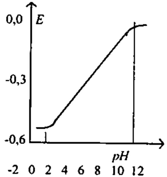
21.2-chizma. Shisha elektrod potensialining pH ga bog'liqligi
