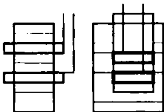
24.11-chizma. Kondensator (sig'im) turidagi elektrolitik bo'g'inning tuzilishi
