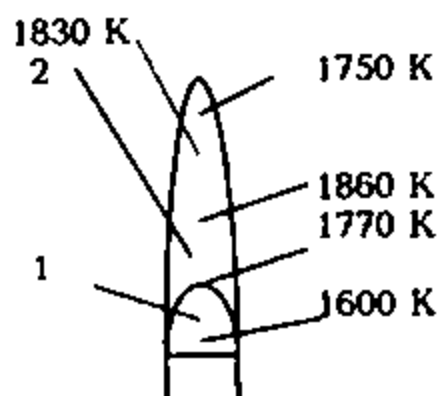
26.1-chizma. Qaldiroq gazning havoda yonish alangasida haroratning taqsimlanishi: 1-qaytarish sohasi; 2-oksidlash sohasi
