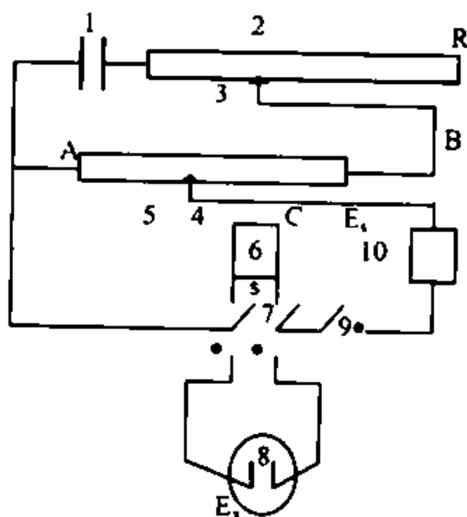
21.11-chizma. Potensialni kompensatsion o'lchash asbobining tuzilishi: 1-akkumulyator; 2-o'zgaruvchan qarshilik; 3,4-sirg'anchiq tutashma; 5-potensiometr; 6-Vestonning normal elementi; 7, 9-kalit; 8-elektrolitik bo'g'in; 10-galvanometr
