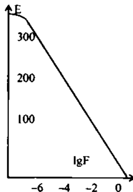
21.4-chizma. Ftorid selektiv elektrodning darajalash chizmasi
