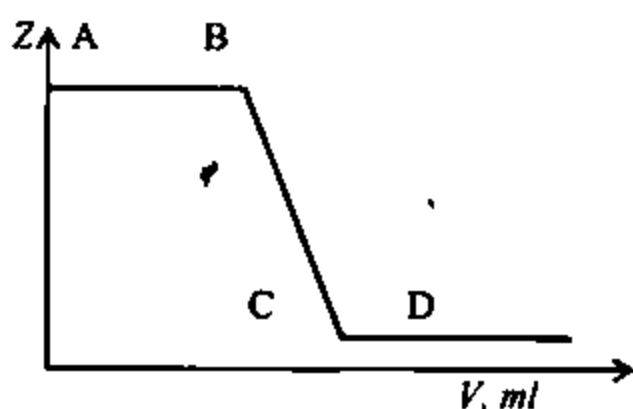
28.8-chizma. Aluminiyni EDTA eritmasi bilan izotopsiz radioaktiv indikator ishtirokida titrlash
