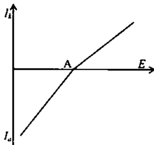
23.6-chizma. Sig'im tokining tomchilaydigan simob elektrodi potensialiga bog'liqligi
