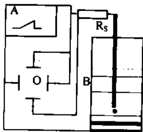
23.13-chizma. Ossillografik polyarografning tuzilishi
