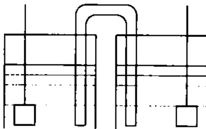
22.18-chizma. Ikki kamerali kulonometrik bo'g'inining tuzilishi
