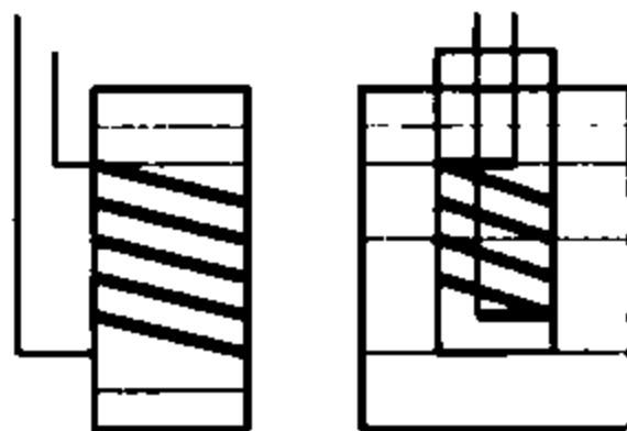
24.12-chizma. Induksion bo'g'inning tuzilishi
