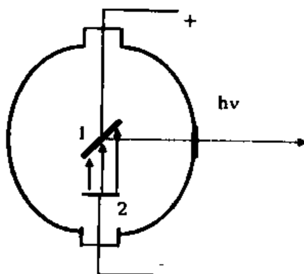
26.8-chizma. Rentgen nayining tuzilishi: 1-anod; 2-katod
