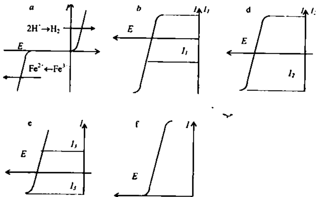
23.19-chizma. Moddaning oksidlovchi bilan titrlanish polyarogrammalari
