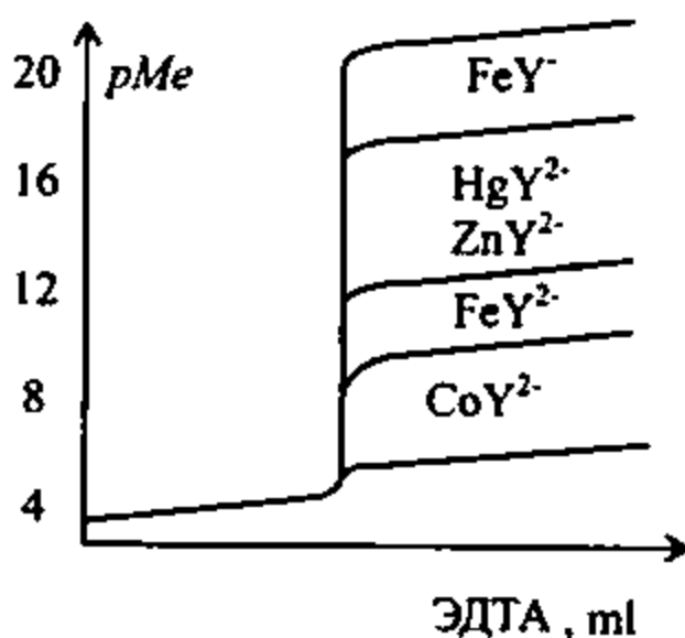
18.3-chizma. 0,01 M kationlarni titrlash egri chizig'i ( pH=6 )
