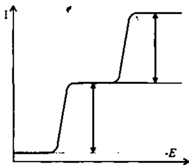
23.8-chizma. Ikkita depolyarizatorli aralashmaning polyarogrammasi balandliklarini aniqlash
