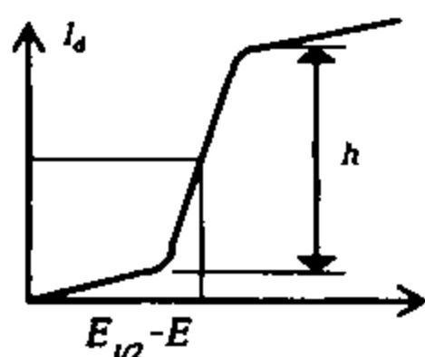
2.1-chizma. Polarogramma
