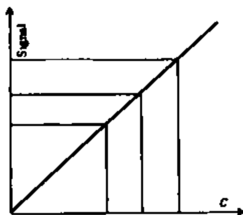
2.4-chizma. Darajalash chizmasi
