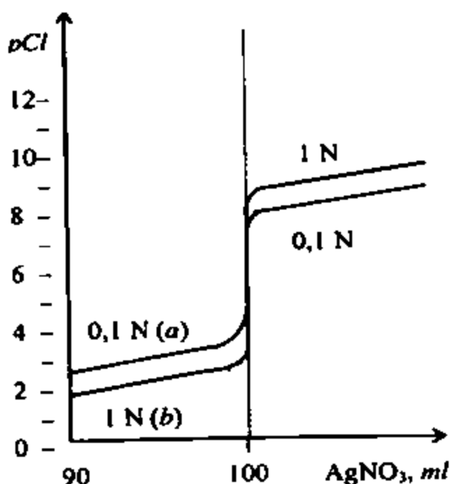
17.1-chizma. Natriy xlorid eritmalarini titrlash egri chiziqlari
