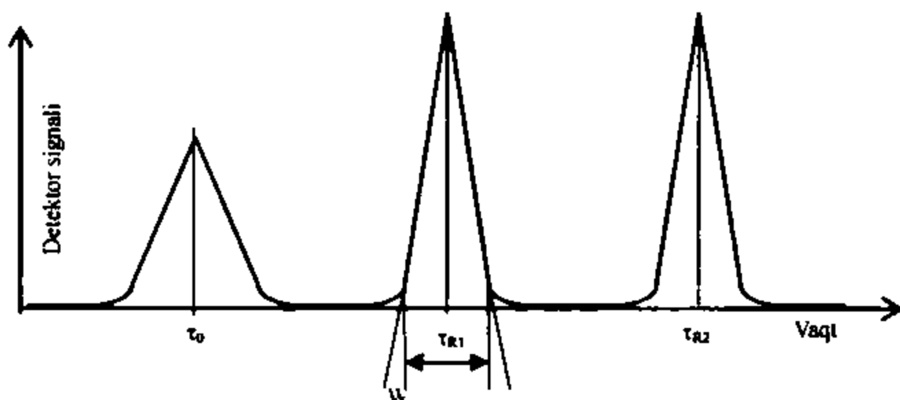
11.2-chizma. Xromatogramma
