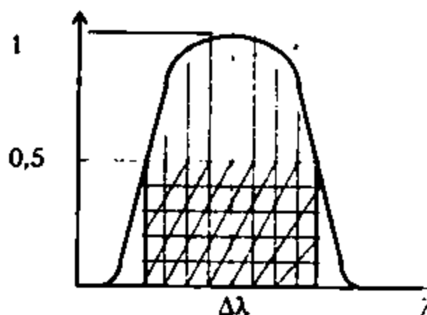
25.5-chizma. Spektr chizig'i va uning yarim kengligi
