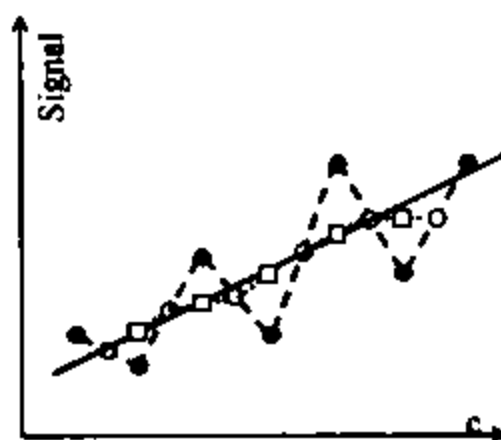
2.5-chizma. Regressiya chizig'i
