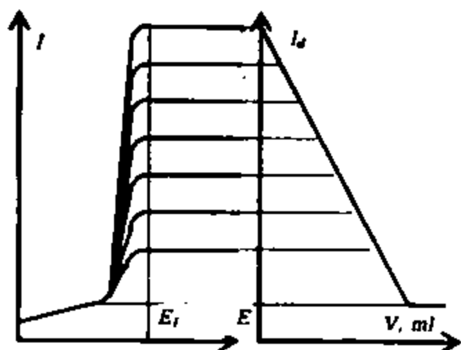
23.17-chizma. Polarografiya bilan amperometrik titrlash orasidagi bog'lanishning chizma tasviri
