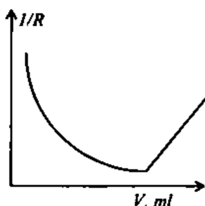
24.5-chizma Monoxlorsirka kislotaning ishqor eritmasi bilan titrlanish egri chizig'i
