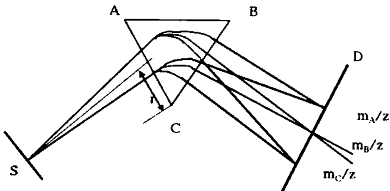
28.4-chizma. Magnit maydonli mass-analizatorning sxemasi
