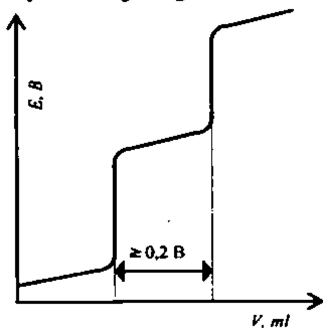
16.3-chizma. Ikki moddani titrlash
