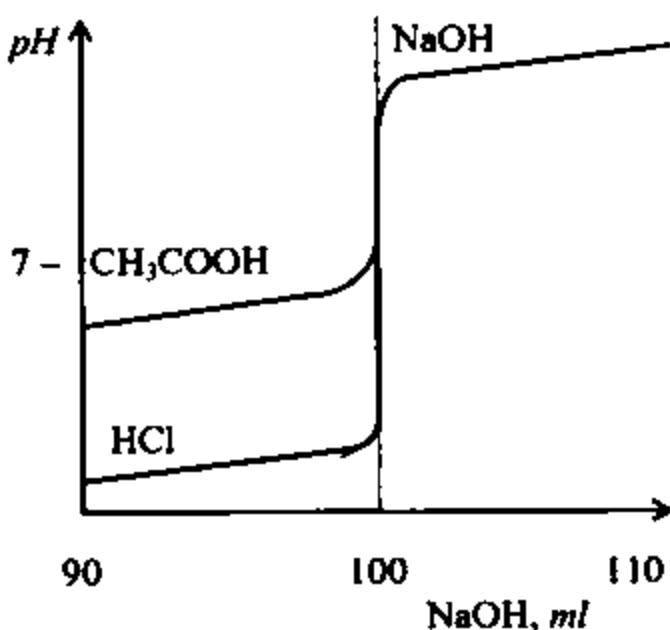
15.5-chizma. Kuchli (HCl) va kuchsiz ( CH_3COOH ) kislotalarni titrlash egri chizilari
