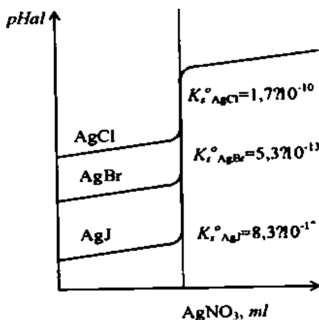
17.2-chizma. Titrlash sakrashiga cho'kmalar eruvchanlik ko'paytmasining ta'siri
