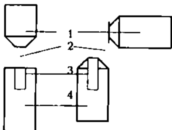
26.3-chizma. Elektr yoyi (uchquni) yordamida ishlaydigan atomizatorning tuzilishi: 1,4-elektrodlar; 2-razryad sohasi; 3-krater
