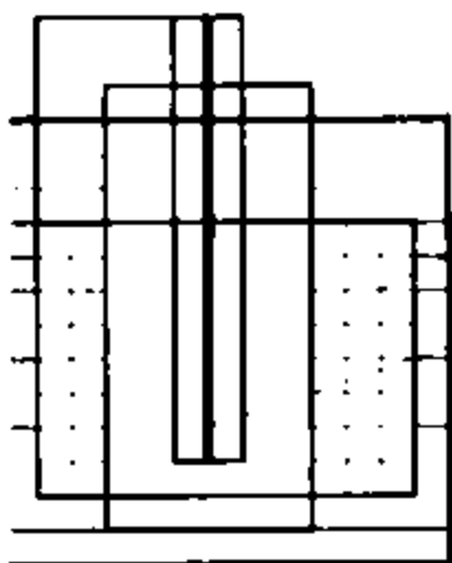
22.22-chizma. Ichki elektroliz asbobining tuzilishi: 1-g'ovak membrana; 2-platina to'ri (silindr); 3-rux elektrodi
