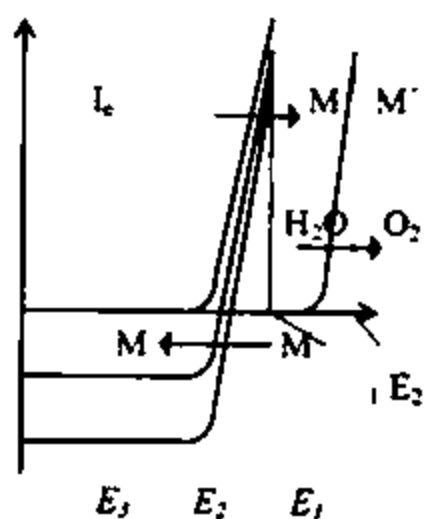
22.10-chizma. Bevosita galvanostatik kulonometriyada ishchi elektrod sirtida elektr aktiv metallni aniqlashda voltamper egri chizmalarining o'zgarishi
