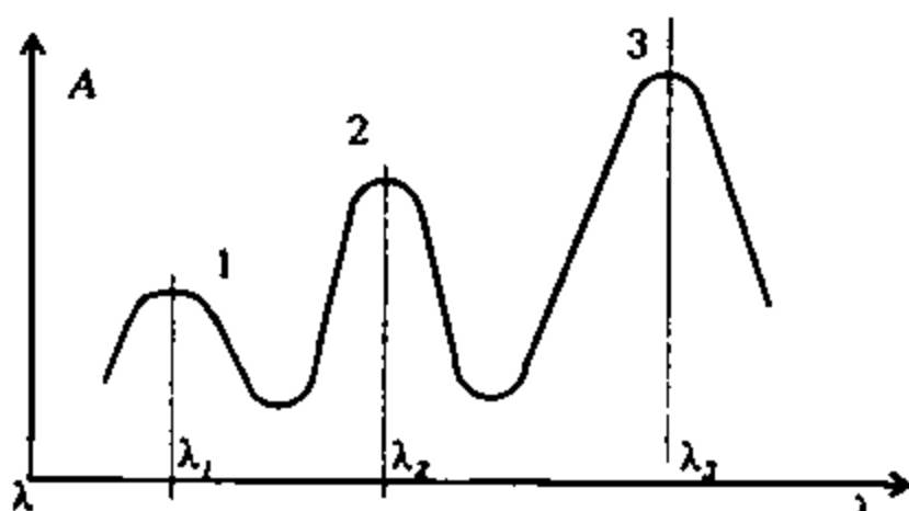
27.3-chizma. Bir necha yutilish yo'lagiga ega bo'lgan moddaning spektri
