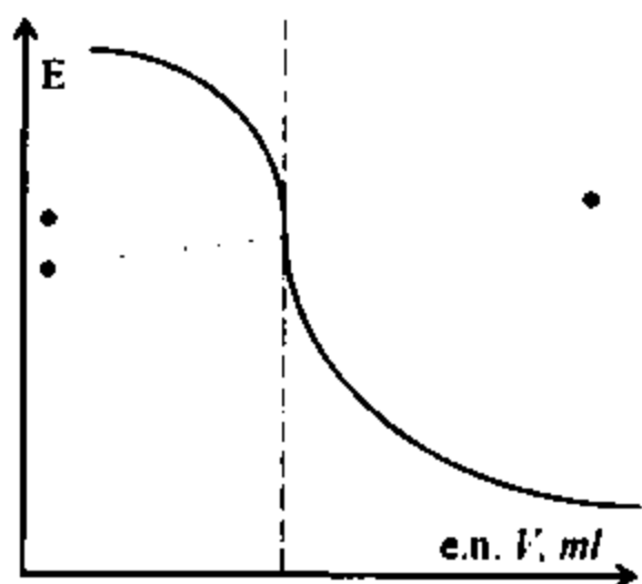
21.8-chizma. Konsentrik yo'lar usuli yordamida titrlashning oxirgi nuqtasini aniqlash
