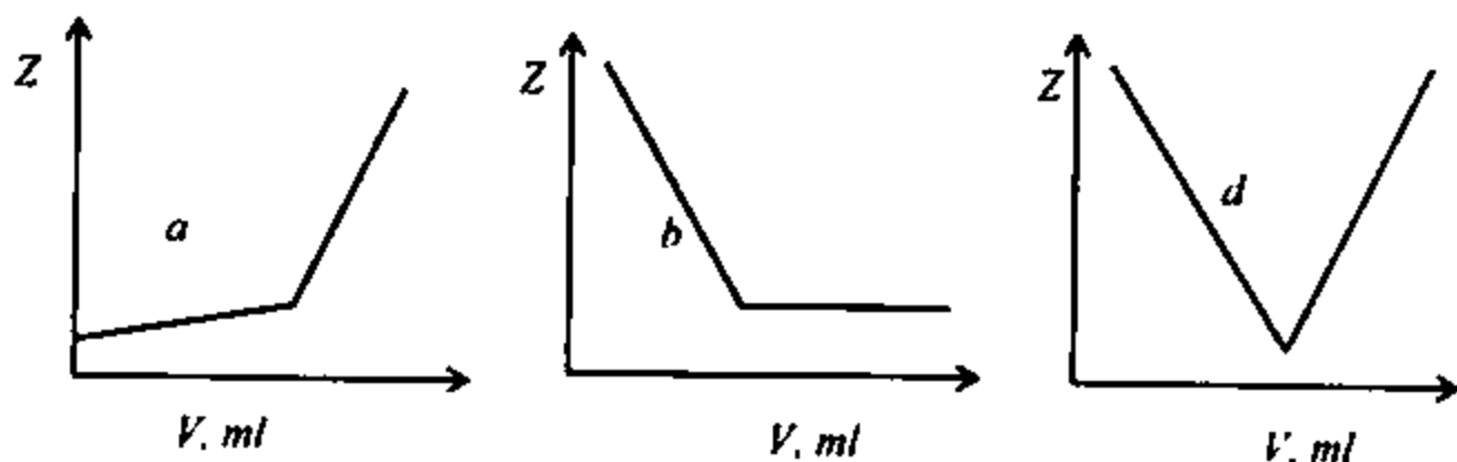
28.6-chizma. Radiometrik titrlash egri chiziqlari:
