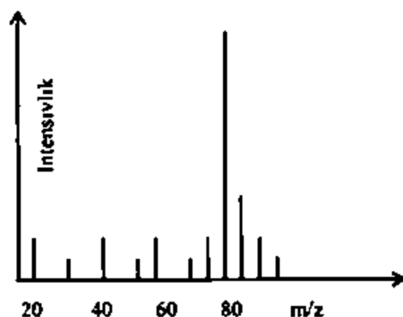
28.2-chizma. Benzolning mass-spektri
