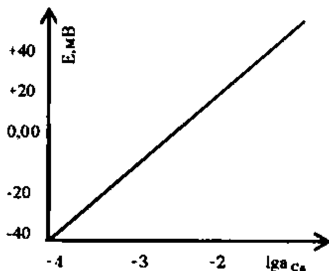
21.6-chizma. Kalsiy selektiv elektrod potentsialining eritmadagi kalsiy ion aktivligiga bog'liqligi
