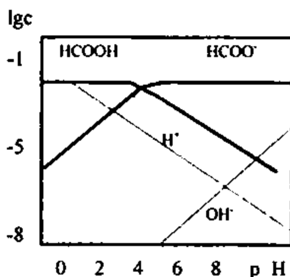
4.2-chizma. Chumoli kislotaning konsentratsion-logarifmik diagrammasi
