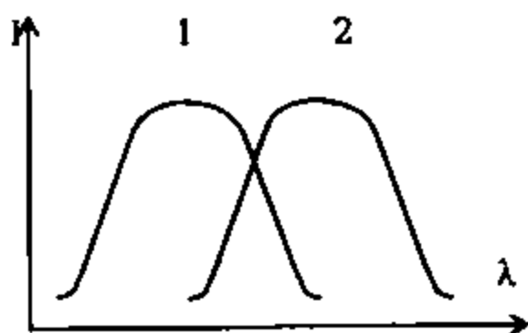
27.8-chizma. Yutilish (1) va lyuminessensiya (2) spektrlarining to'lqin uzunliklari
