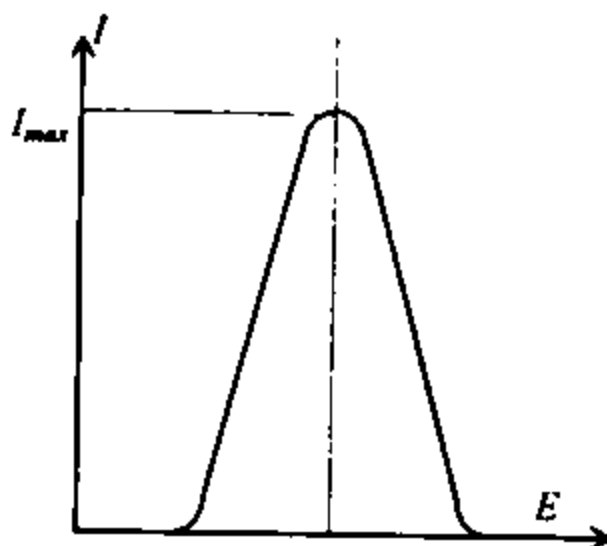
23.16-chizma. Kvadrat to'liqinli polyarografiyaning voltamper egri chizig'i
