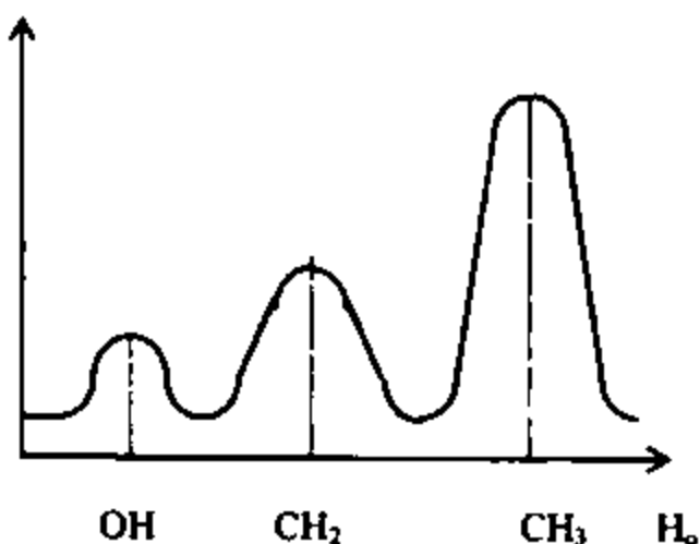
28.5-chizma. Etanolning YAMR spektri
