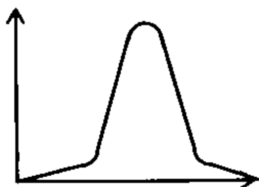
2.2-chizma. Taqsimot chizmasi
