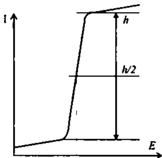
23.7-chizma. Polyarografik to'liqining balandligi va yarim to'liqin potensialini aniqlash
