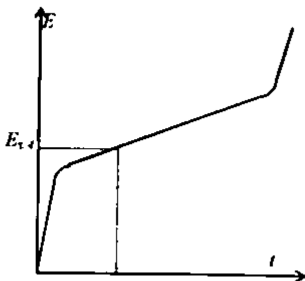
23.15-chizma. Xronopotensiogramma
