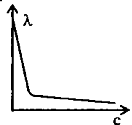
24.3-chizma. Molekulyar elektr o'tkazuvchanlikning konsentratsiyaga bog'liqligi
