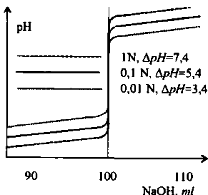
15.3-chizma. Eritma pH sakrashining konsentratsiyaga bog'liqligi
