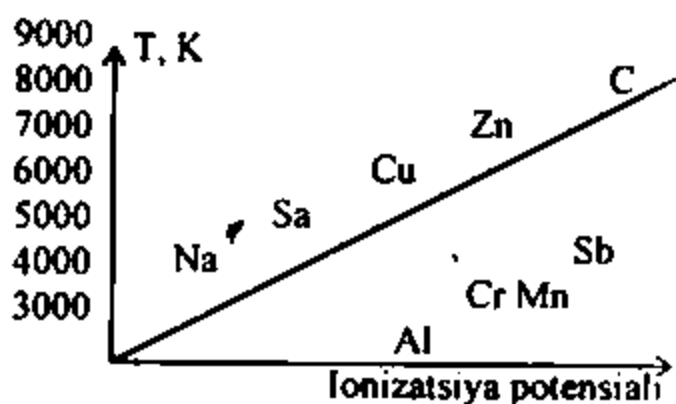
26.4-chizma. Turli ionizatsiya potentsialiga ega bo'lgan moddalarni kiritganda yoy haroratining o'zgarishi
