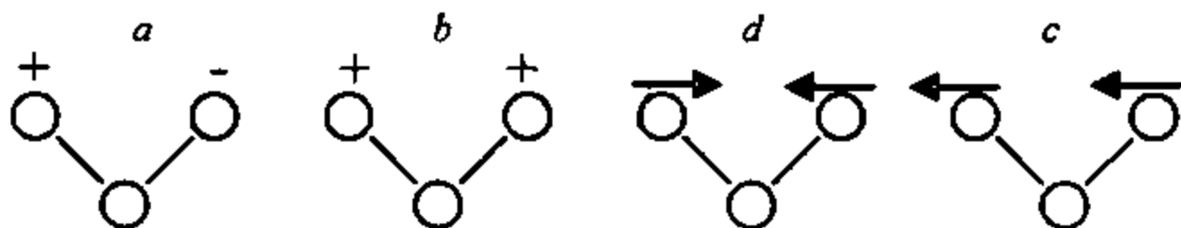
25.8-chizma. Deformatsion tebranishlarning turlari:
