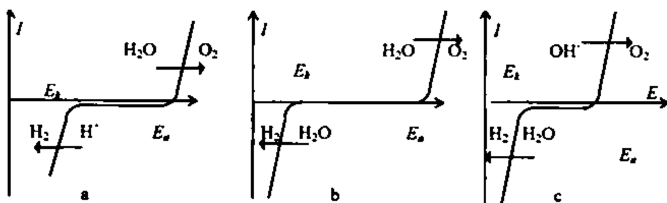
20.7-chizma. Suvning turli muhitlardagi voltamper egri chiziqlari:
