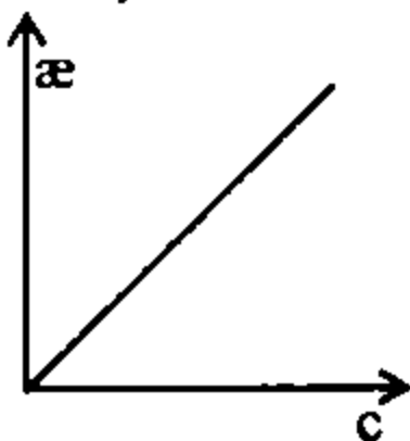
24.1-chizma. Solishtirma elektr o'tkazuvchanlikning konsentratsiyaga bog'liqligi
