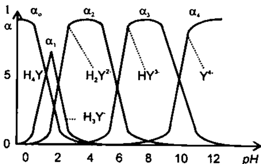
18.1-chizma. EDTA eritmasi tarkibining pH qiymatiga bog'liqligi
