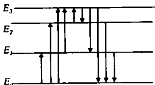
25.2-chizma. Atomlarning energetik holatlaridagi o'tishlar:
