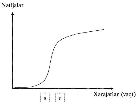
4.1-chizma. S ko'rinishdagi egri chiziq.
