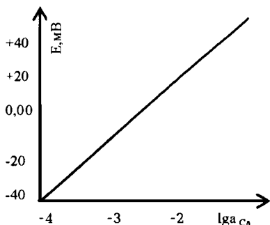
21.6-chizma. Kalsiy selektiv elektrod potentsialining eritmada kalsiy ion aktivligiga bog'liqligi
