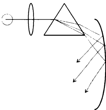
25.9-chizma. Prizma yordamida monoxromatlash
