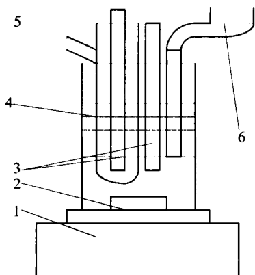
21.10-chizma. Potentsiometrik differensial titrlash uchun qurilma.
