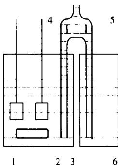
22.20-chizma. Titrantni tashqi generatsiya qilish usuli bilan titrlash bo'g'inining tuzilishi:
