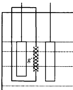
22.7-chizma. Titratsion kulonometrning tuzilishi
