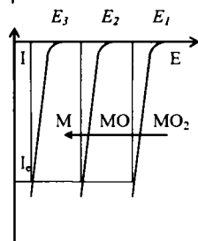
22.11-chizma. Bevosita galvanostatik kulonometriyada elektr aktiv metall oksidining ( MO_2 ) ketma-ket qaytarilishida volt-ampere egri chizig'ining o'zgarishi
