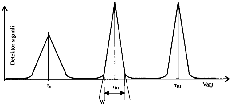
11.2-chizma. Xromatogramma
