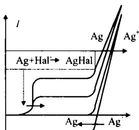
22.17-chizma. Galogenidlarni elektr generatsiya qilingan Ag^+ bilan titrlashda voltamper egri chizig'ining o'zgarishi
