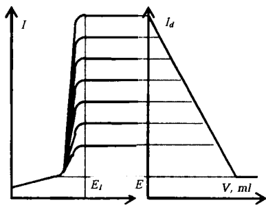
23.17-chizma. Polyarografiya bilan amperometrik titrlash orasidagi bog'lanishning chizma tasviri
