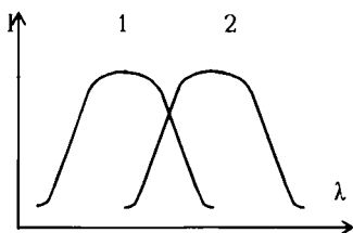
27.8-chizma. Yutilish (1) va lyuminessensiya (2) spektrlarining to'lqin uzunliklari
