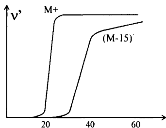
28.1-chizma. Atseton molekulasini nisbiy chastotasining ( v' ) elektron energiyasiga bog'liqligi
