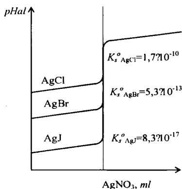
17.2-chizma. Titrlash sakrashiga cho'kmal eruvchanlik ko'paytmasining ta'siri
