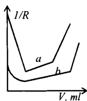
24.8-chizma. Ikki negizli kislotalarni ishqor eritmasi bilan titrlash: a-xromat kislota; b-malein kislota
