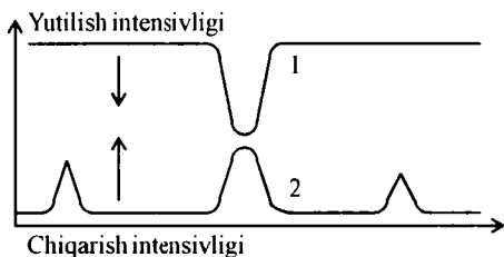
26.5-chizma. Atom-absorbsion spektroskopiyada chiqarish va yutilish spektrlari:
