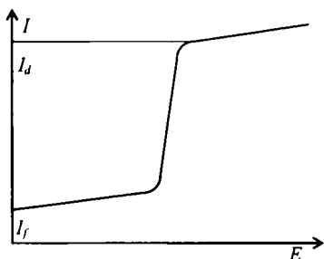
22.3-chizma. Voltamper egri chizig'i
