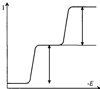
23.8-chizma. Ikkita depolyarizatorli aralashmaning polarogrammasi balandliklarini aniqlash
