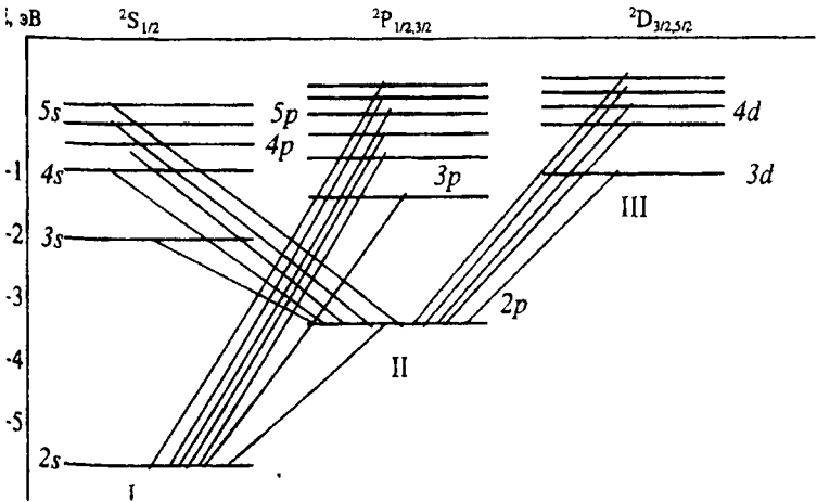
25.6-chizma. Litiy atomi energetik sathlarining sxemasi:
