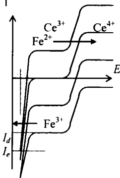
22.14-chizma. Seriy (IV) ionini elektr generatsiya qilingan temir (II) ionni yordamida titrlash jarayonida voltamper egri chizig'ining o'zgarishi
