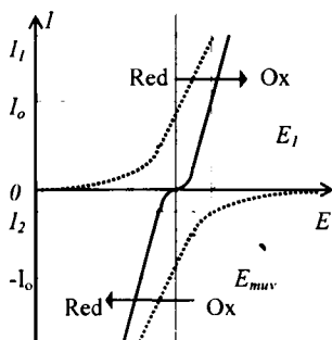
20.6-chizma. Qaytar sistemaning voltamper egri chizig'i
