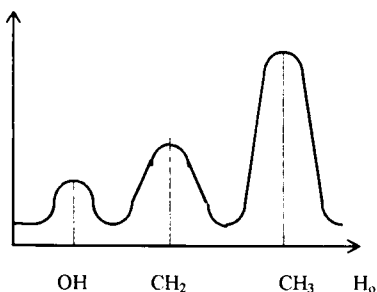
28.5-chizma. Etanolning YAMR spektri
