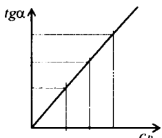
19.1-chizma. Tangenslar usuli bo'yicha aniqlash
