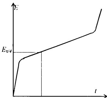
23.15-chizma. Xronopotensiogramma
