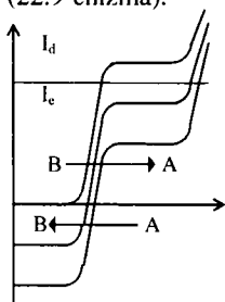
22.9-chizma. Bevosita galvanostatik kulonometriyada modda konsentratsiyasining o'zgarishi bilan voltamper egri chiziqlarining o'zgarishi
