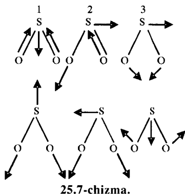
SO 2 molekulasidagi tebranishlar
