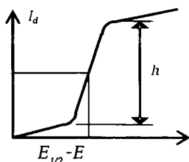
2.1-chizma. Polarogramma
