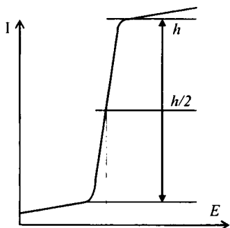
23.7-chizma. Polarografik to'liqning balandligi va yarim to'liq potensialini aniqlash
