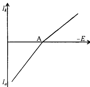
23.6-chizma. Sig'im tokning tomchilaydigan simob elektrod potentsialiga bog'liqligi
