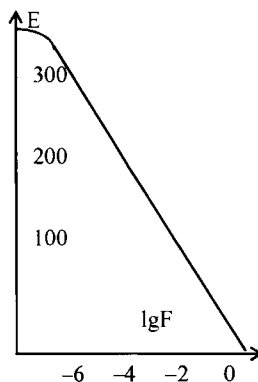
21.4-chizma. Ftorid selektiv elektrodning darajalash chizmasi
