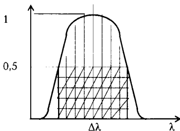
25.5-chizma. Spektr chizig'i va uning yarim kengligi
