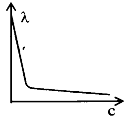
24.3-chizma. Molekulyar elektr o'tkazuvchanlikning konsentratsiyaga bog'liqligi
