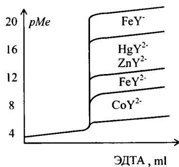
18.3-chizma. 0,01 M kationlarni titrlash egri chizig'i ( pH=6 )
