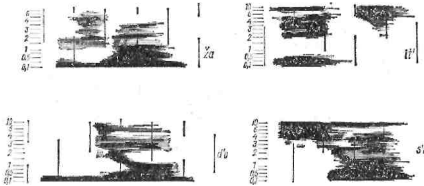
Рис. 2. Спектрограммы слогов, взятых из слов русского языка. Цифры на шкале обозначают килогерцы
