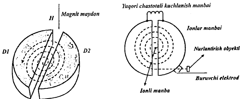
5.1-rasm. Siklotron. Siklotronida ionlar harakati.
