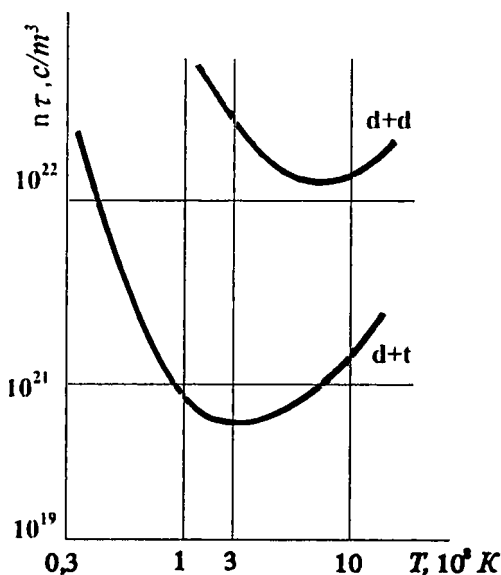
5.15-rasm. Deyteriy-tritii, deyteriy-deyteriy reaksiyalari uchun plazmani ushlash parametrining temperaturaga bog‘liqligi.
