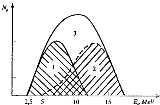
5.10-rasm. Indiy yadrosidan uchib chiqqan fotoprotonlar spektri: 1 va 2-bug'lanish va bevosita fotoeffekt mexanizmlarga taalluqli nazariy egri chiziqlar; N_p – nisbiy intensivlik.
